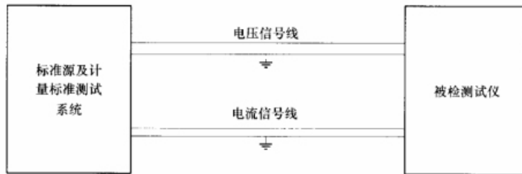
图 A.1 校验接线
