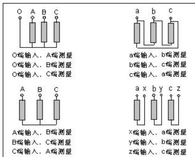
图2 变压器的几种常用检测接线方式
