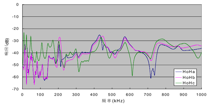
图B.8 SSSO3-120000/220变压器高压绕组变形时的幅频响应曲线
