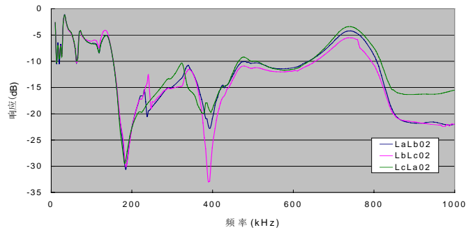
图 B.1 b) SFPSZ7-120000/220 变压器低压绕组修复后的幅频响应曲线
