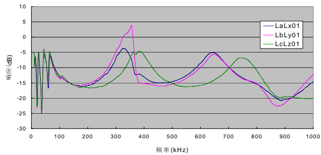
图 B.2 a) SFPSZ7-150000/220 变压器低压绕组变形时的幅频响应曲线
