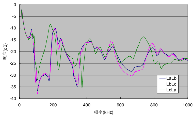
图4 某台变压器遭受突发短路后三相低压绕组的幅频响应特性曲线
