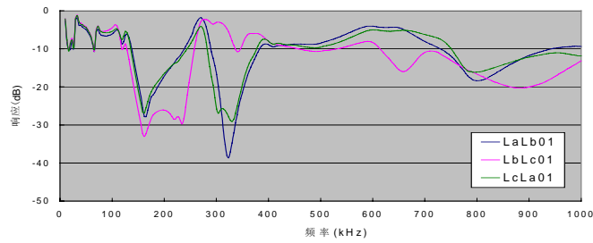
图 B.1 a) SFPSZ7-120000/220 变压器低压绕组变形时的幅频响应曲线
