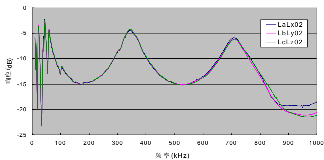
图 B.2 b) SFPSZ7-150000/220 变压器低压绕组修复后的幅频响应曲线
