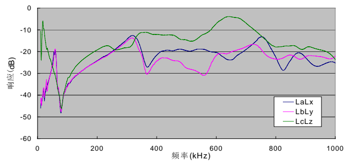
图B.5 SF9-31500/110变压器低压绕组变形时的幅频响应曲线
