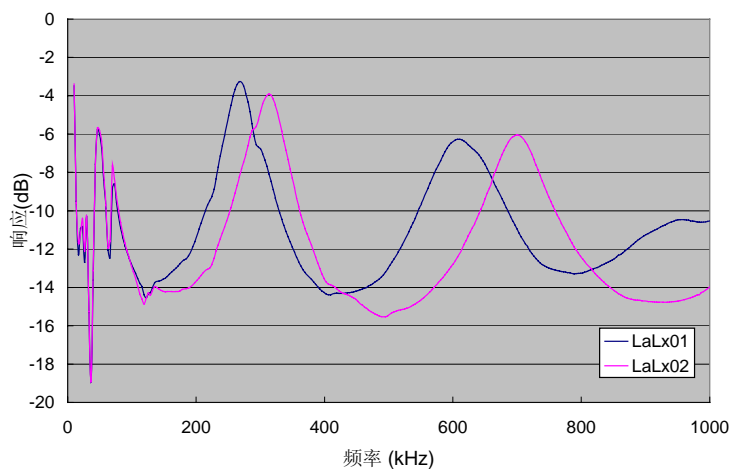
图3 某台变压器在遭受短路电流冲击前后的幅频响应特性曲线
