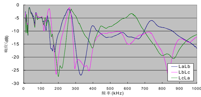
图B.4 SFPSZ7-150000/220变压器低压绕组变形时的幅频响应曲线
