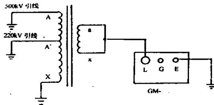
500kV 电力变压器低压绕组绝缘测试接线图
