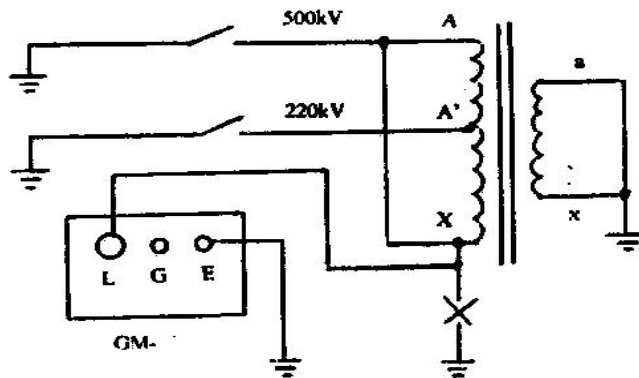
500kV 电力变压器高压绕组绝缘测试接线图
