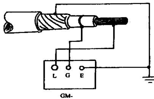
屏蔽电缆绝缘测试接线图
